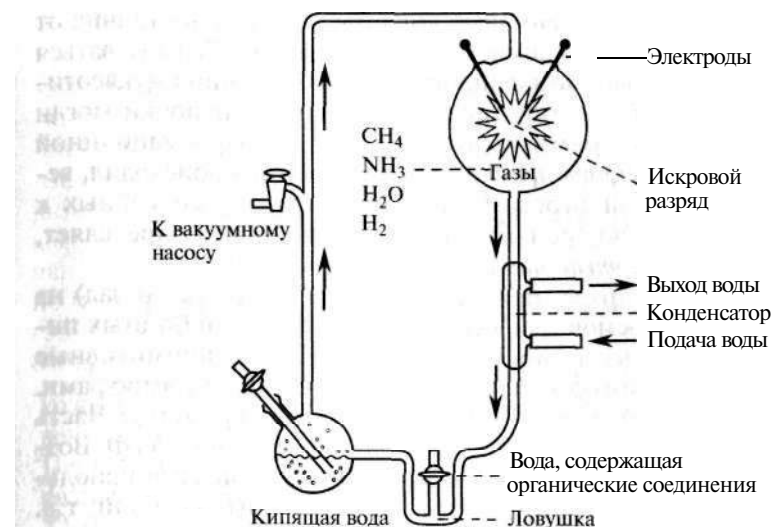
Рис. 4.3. Аппарат Миллера
